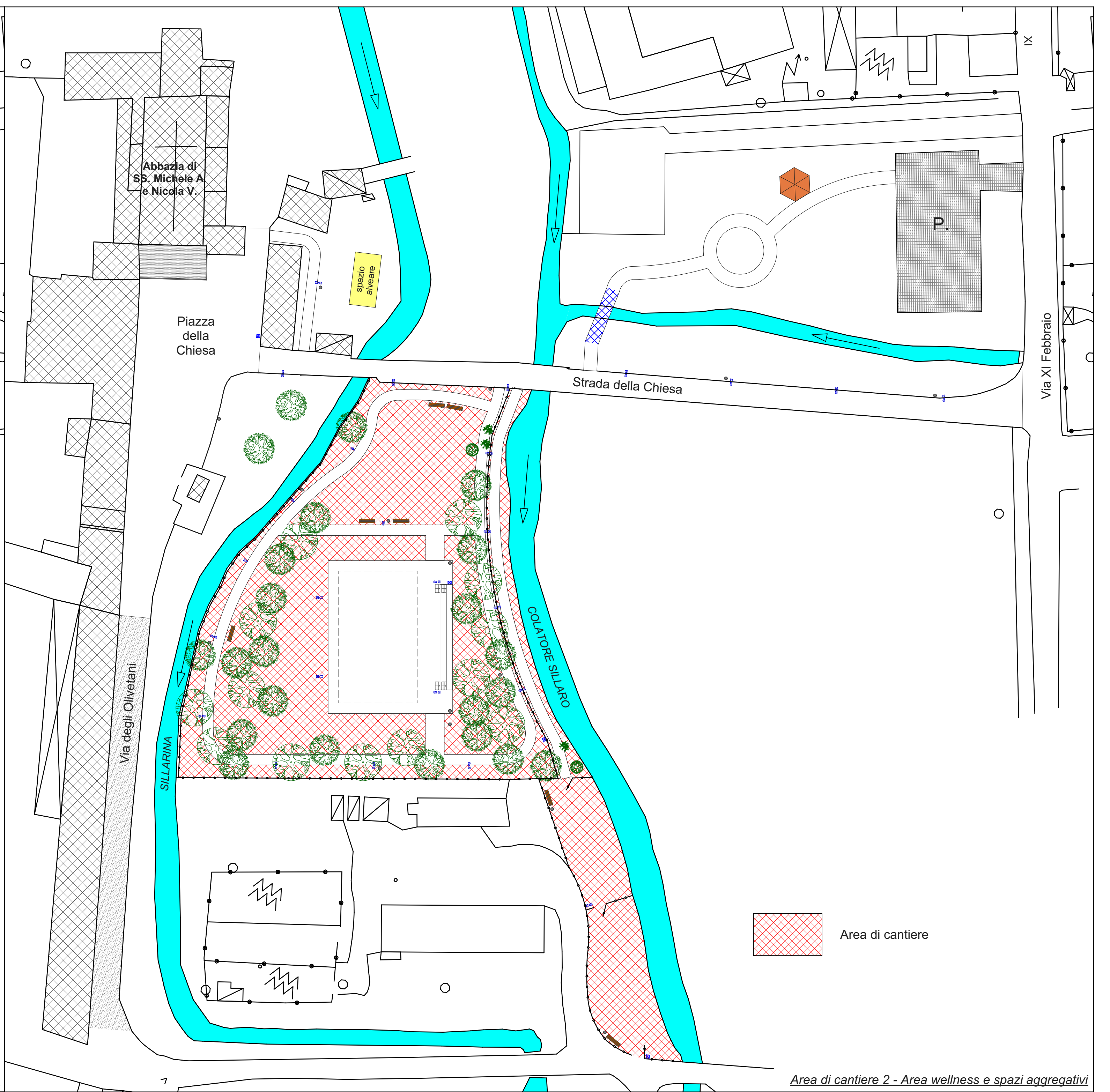
Area di cantiere 2 - Area wellness e spazi aggregativi
